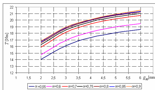
Rys. 3. Zależność momentu od grubości magnesu
