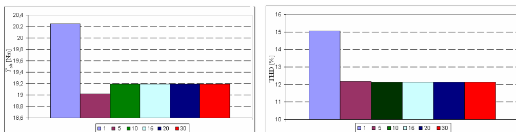
Rys. 4. Porównanie wartości momentu, współczynnika THD oraz objętości magnesów w 30 pokoleniach Fig. 4. Comparison of torque, THD factor and magnet volume during optimization process
