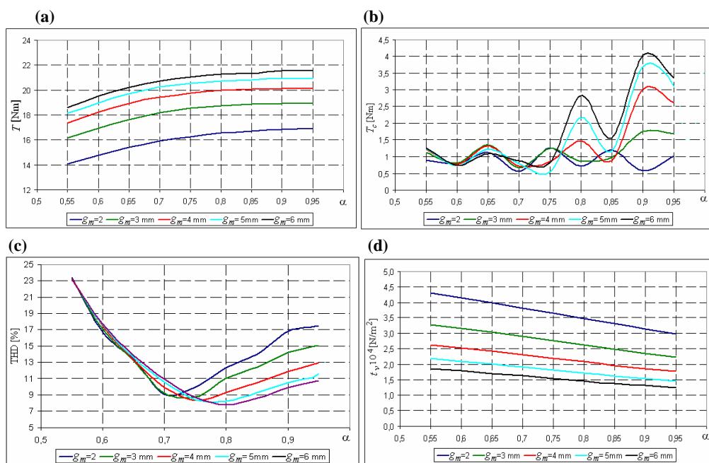
Rys. 2. Wpływ zmiennych g_m i \alpha na parametry T , T_c , THD oraz t_v Fig. 2. The influence of g_m and \alpha on parameters T , T_c , THD and t_v
